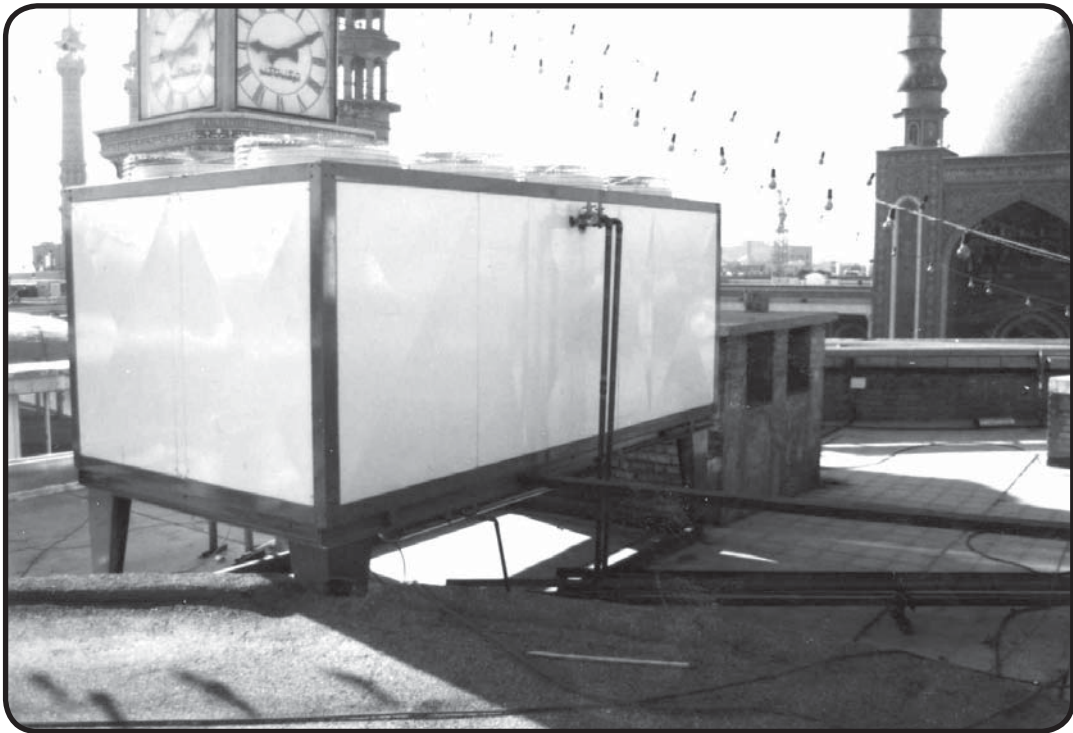
موتورخانه حرارتی و موتورخانه آبردکن مرکزی حرم مطهر یک دستگاه منبع ذخیره انبساط آبردکن مرکزی، مستقر در پشت بام مسجد اعظم
