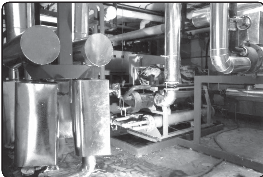
موتورخانه حرارتی و موتورخانه آب سردکن مرکزی حرم مطهر موتورخانه آب سردکن مرکزی مستقر در زیرزمین کتابخانه
