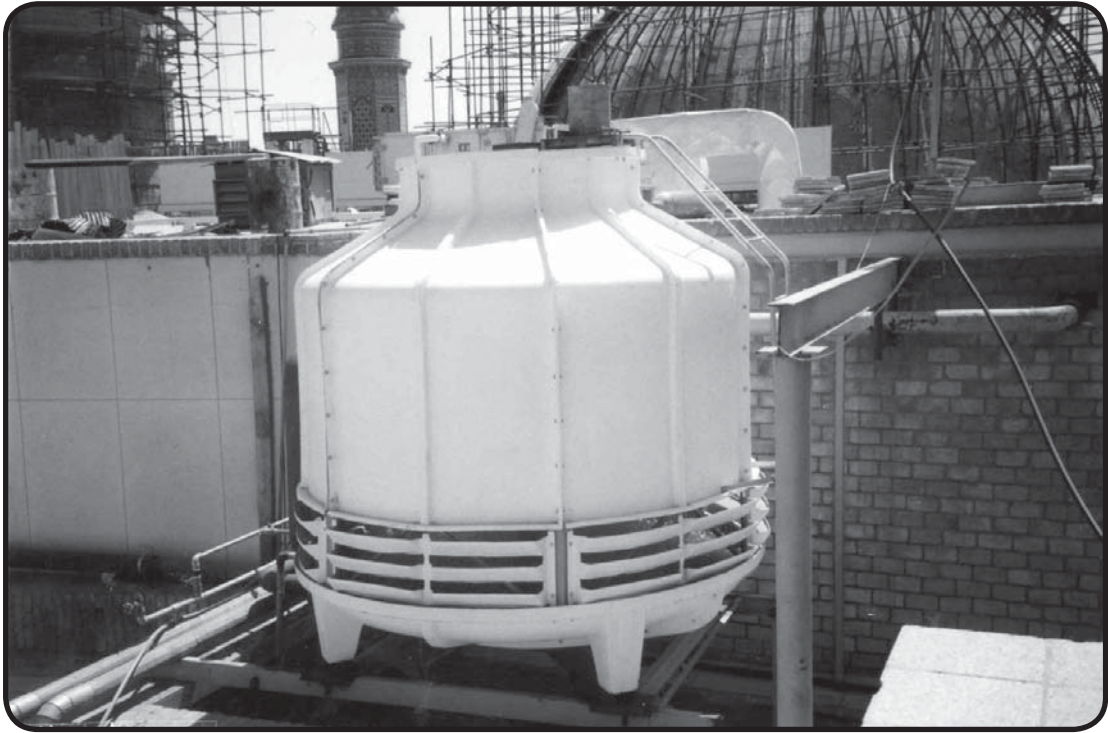
تاسیسات سرمایشی و گرمایشی حرم مطهر شامل برج خنک کننده، منبع و موتورخانه
