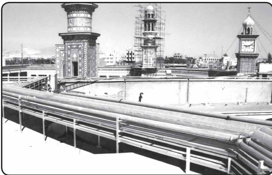
کانال کشی و داکت کشی جهت انتقال کابلها در پشت بام حرم مطهر، دهه ۱۳۸۰
