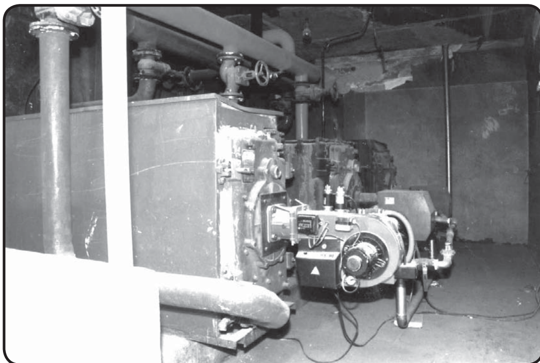
موتورخانه حرارتی و موتورخانه آب سردکن مرکزی حرم مطهر موتورخانه حرارتی ساختمان کتابخانه، در مانگاه و مهمانسرای شامل چهار دستگاه دیک ۴۰۰ ده پر
