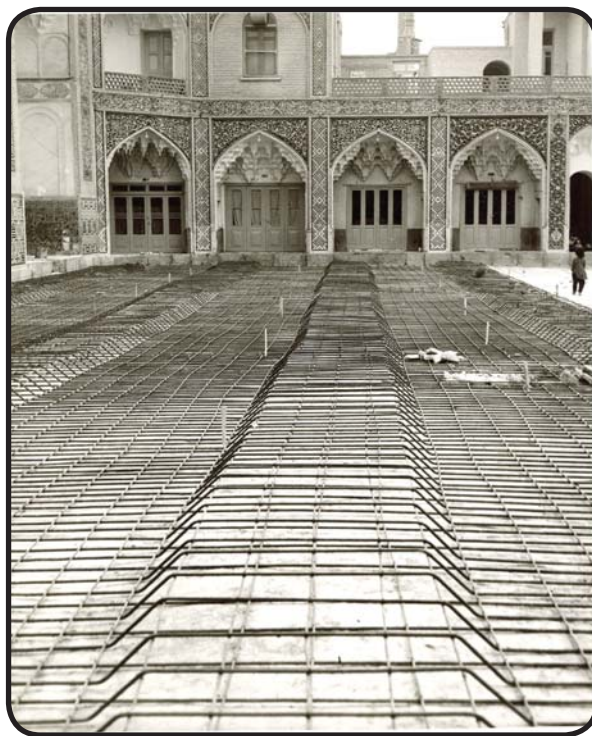
بتن ریزی کف صحن عتیق، سال ۱۳۴۹
