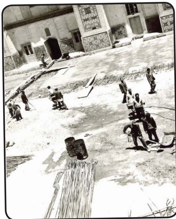
بتن ریزی کف صحن عتیق، سال ۱۳۴۹
