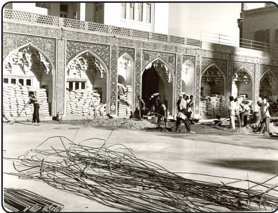
بتن ریزی کف صحن عتیق، سال ۱۳۴۹
